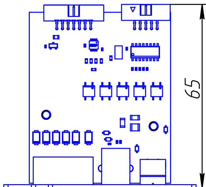
Рисунок 1.2 – Габаритные размеры изделия
